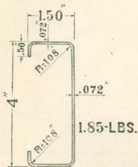
4"—1.85 lb. Channel Stud
