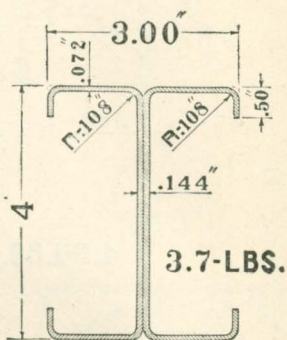
4"—3.7 lb. I Stud
